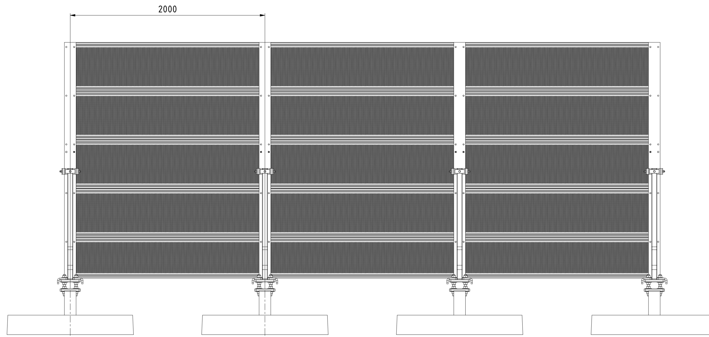
TRAFIKSIDA ( 1 : 20 )
