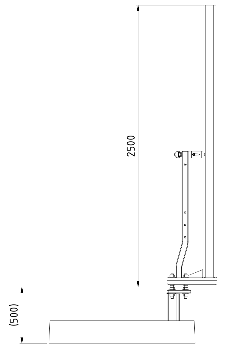
SIDOVY ( 1 : 20 )
